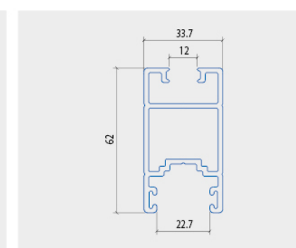
THANH ĐỨNG CÁN H
