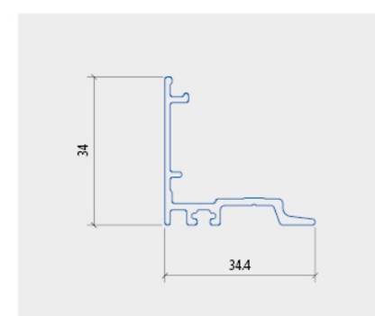
NỆM CẢNH CỬA TRƯỢT
