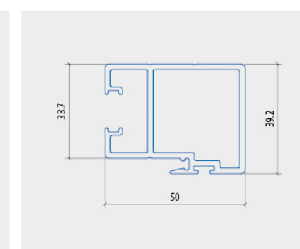
THANH ĐỨNG CÁN H MÓC
