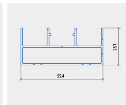
ĐỨNG KB LÙA 1 RAY
