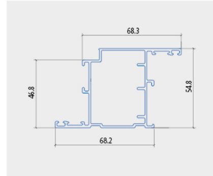
CÁNH CỬA ĐI MỞ TRONG
