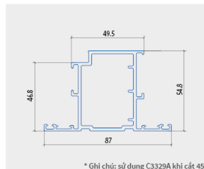
CÁNH CỬA ĐI MỞ NGOÀI
