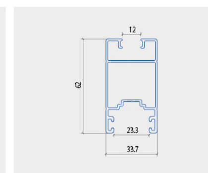
THANH ĐỨNG CÁNH
