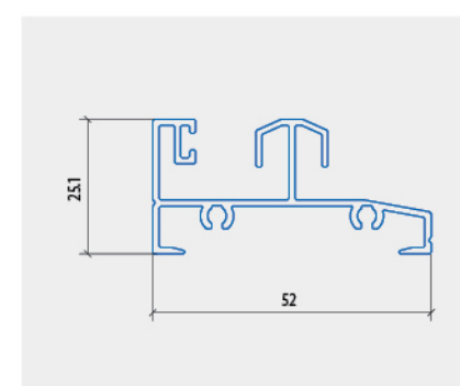
NGANG RAY DƯỚI LÙA 1 RAY
