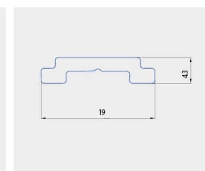
THANH TRUYỀN KHÓA ĐA ĐIỂM
