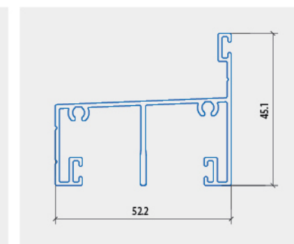
NGANG RAY TRÊN LÙA 1 RAY
