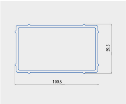
NÒNG NỐI MD651
