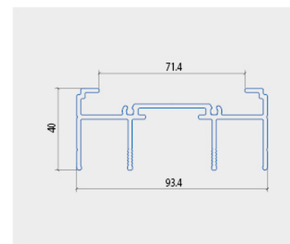
RAY TRÊN
