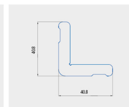
KE LIÊN KẾT CHO CÁNH VÀ KHUNG BAO CỬA BẬT
