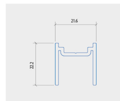
NỆM KÍNH HỘP CỬA TRƯỢT
