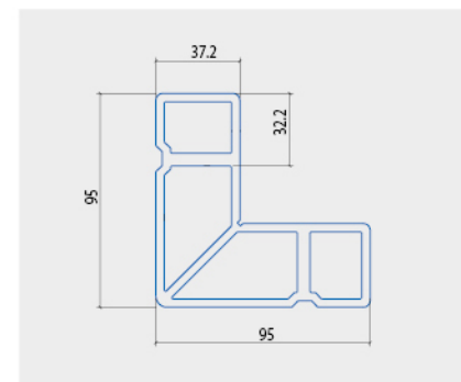
KE GÓC
