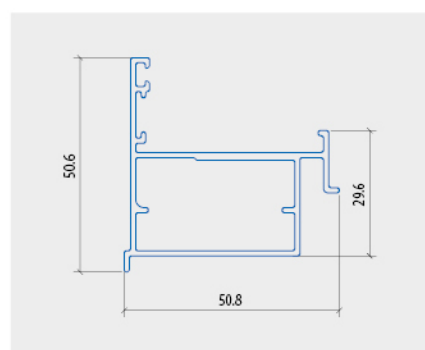
NỆP CHUYỂN HƯỚNG CHIẾU MỞ
