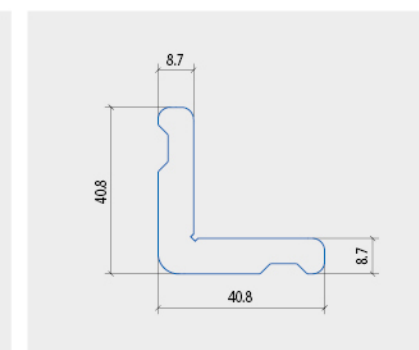
KE GÓC CỬA SỔ
