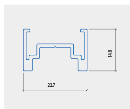
NẾP CHO KÍNH HỘP CỬA TRƯỢT
