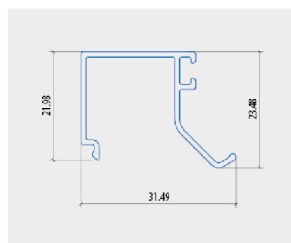
NỆP KÍNH
