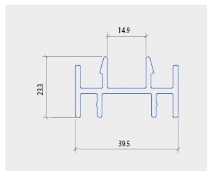
THANH ỚP ĐỐI ĐẦU 4 CÁNH
