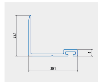
ỐP ĐỨNG CÁNH LÙA 1 RAY
