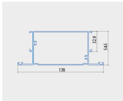
NGANG CÁNH DƯỚI CẮT 90 ĐỘ CỬA ĐI
