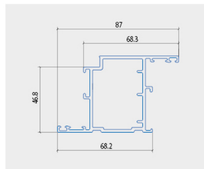
CÁNH CỬA ĐI MỞ TRONG
