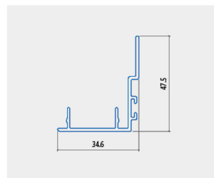
NẾP GÀI CỬA TRƯỢT 55
