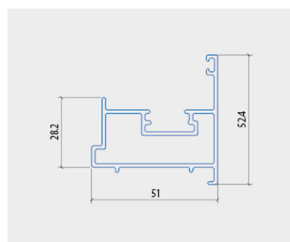
ĐỖ ĐỘNG CỬA SỔ
