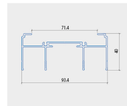
RAY TRÊN
