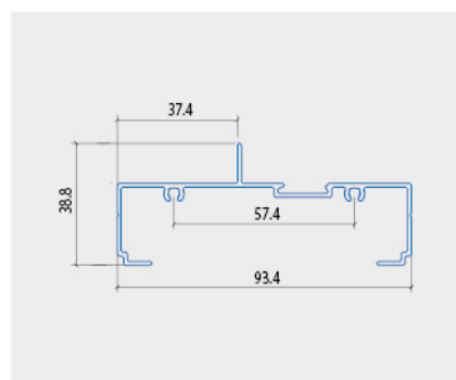
KHUNG BAO VÁCH KÍNH
