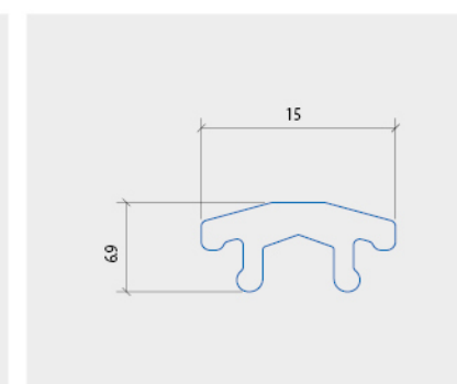
RĂNG THANH TRUYỀN CỬA TRƯỢT
