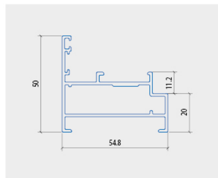
KHUNG BAO CỬA SỔ
