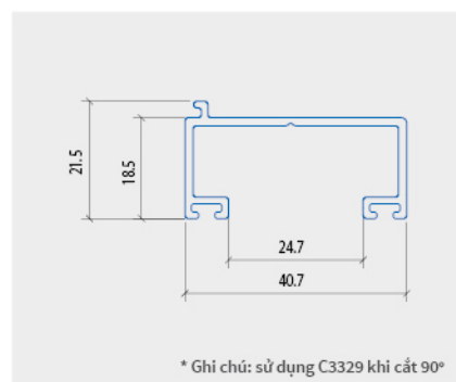
ỐP CHÂN CỬA ĐI
