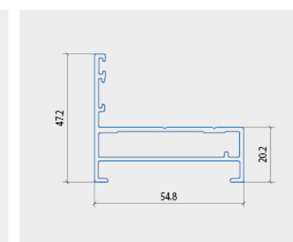
KHUNG BAO CỬA MẶT DỰNG
