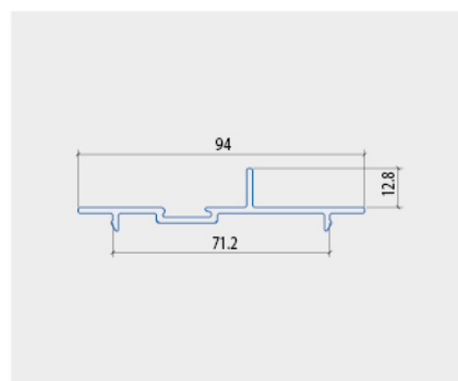
ỐP NẸP NGANG KHUNG BAO
