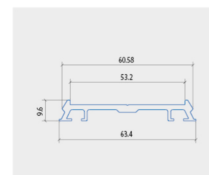
NẾP KHUNG NHÔM NỔI
