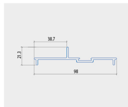
ỐP NẸP ĐỨNG KHUNG BAO ĐỨNG
