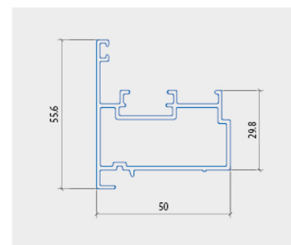
ĐỒ ĐỘNG DỪNG CHUNG (Mã dùng riêng)
