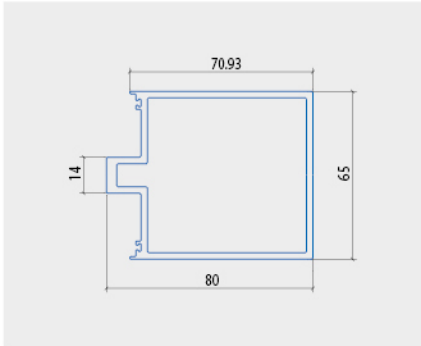
THANH ĐỨNG 80*65
