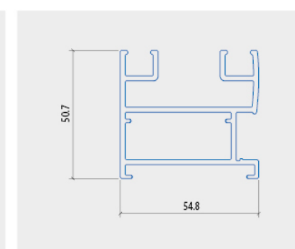
KHUNG BAO CỬA TRƯỢT
