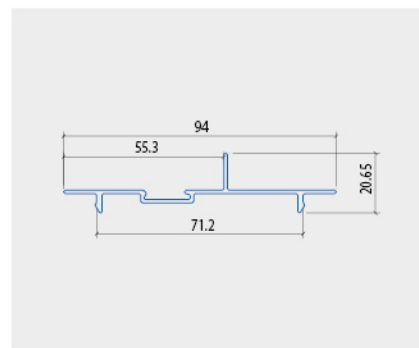
ỐP NẸP NGANG KHUNG BAO
