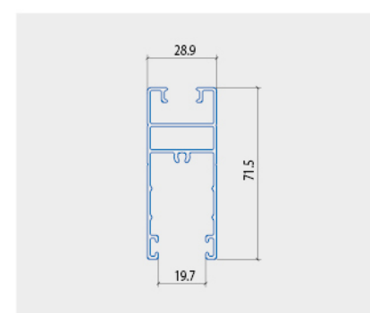
THANH NGANG CÁN H DƯỚI
