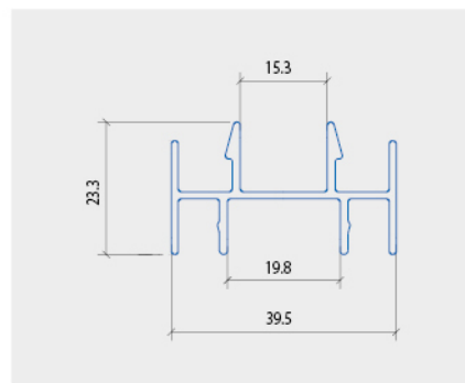
THANH ỐP ĐỐI ĐẦU 4 CẠNH
