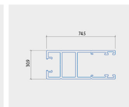
KHUNG CẢNH CỬA TRƯỢT
