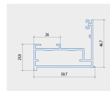
CÁNH CỬA BẬT MẶT DỰNG
