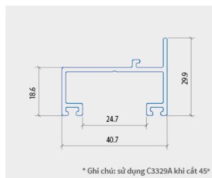
ỐP CHÂN CỬA ĐI
