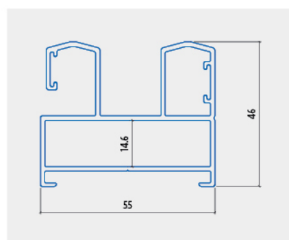
KHUNG BAO CỬA TRƯỢT 55
