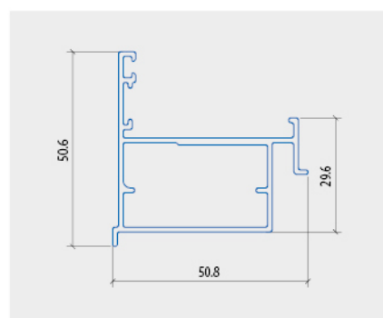
NỆP CHUYỂN HƯỚNG CHIỀU MỞ
