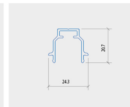
ỐP ĐỐI ĐẦU 4 CẢNH CỬA TRƯỢT
