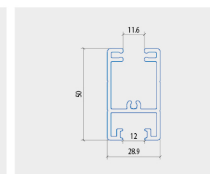
NGANG CÁN H TRÊN
