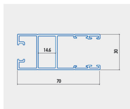
KHUNG CÁNH CỬA TRƯỢT 55
