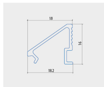
NẸP KÍNH
