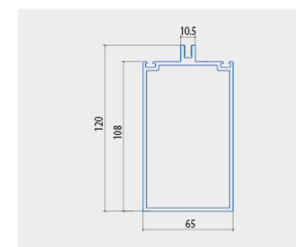
THANH ĐỨNG 65*120
