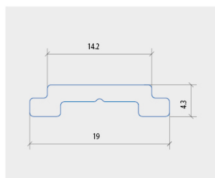
THANH TRUYỀN ĐỘNG
