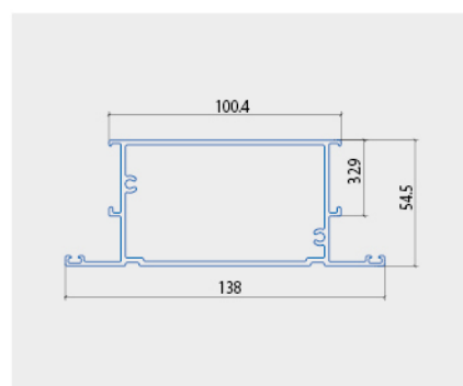
CÁNH CỬA ĐI NGANG DƯỚI
