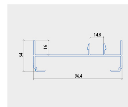
KHUNG BAO ĐỨNG
