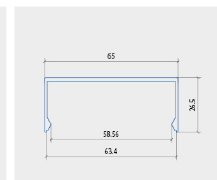
NẮP ĐÁY KHUNG NHÔM NỔI
