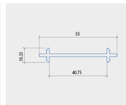
NỆP NỐI KHUNG
