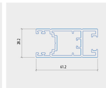
KHUNG CẢNH CỬA TRƯỢT
