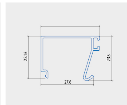
NỆP KÍNH
