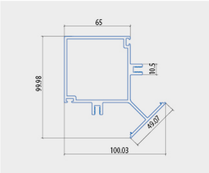
THANH ĐỨNG GÓC 90 ĐỘ
