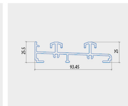
RAY DƯỚI
