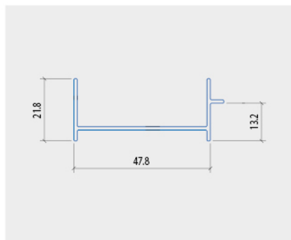
KHUNG BAO LÁ SÁCH
