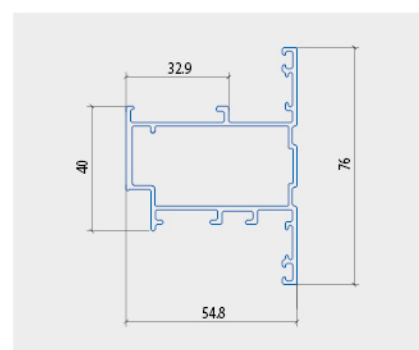
CÁNH CỬA SỔ (Mã dùng riêng)
