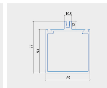
NGANG NHỎ 65*77
