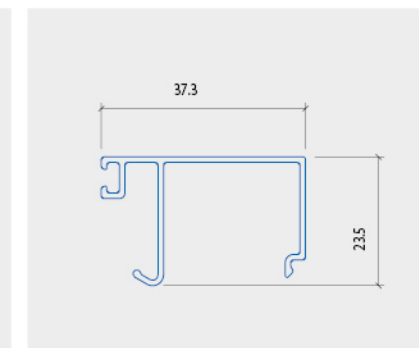
NỆP KÍNH KHUNG CÁNH
