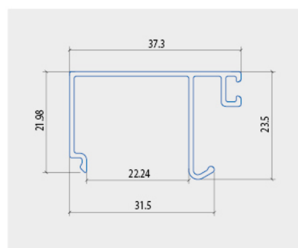
NỆP KÍNH KHUNG CÁNH
