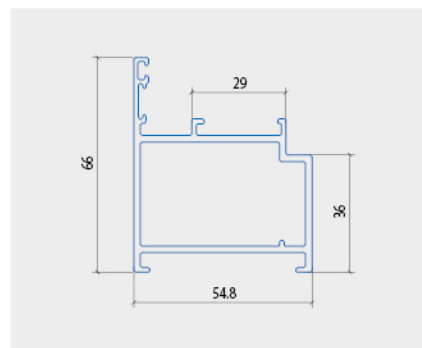
KHUNG BAO CỬA ĐI
