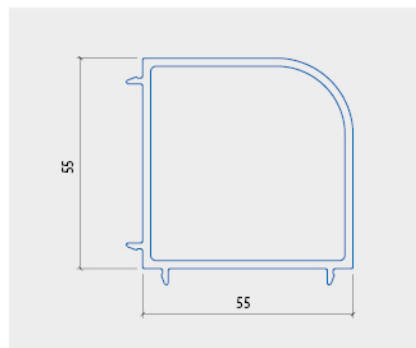
ỐP GÓC 90°
