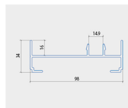
KHUNG BAO ĐỪNG
