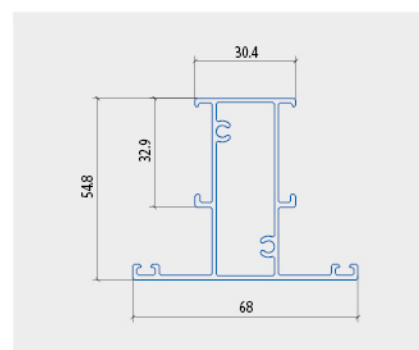
ĐỖ CHỨT CHO CÁNH
