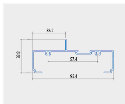
KHUNG BAO VÁCH KÍNH
